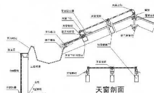
天窗剖面
